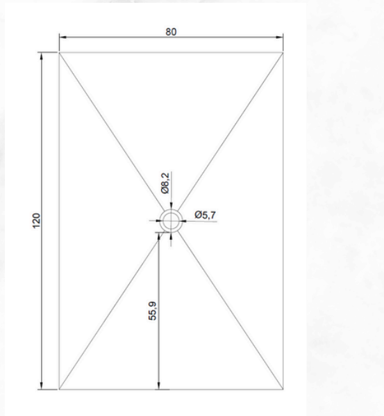
COD.PD_2 PIATTO DOCCIA 120X80
