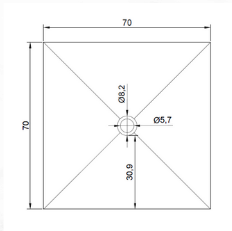
COD.PD_1 PIATTO DOCCIA 70X70
