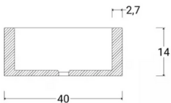
COD.LE 1 LAVABO 40X40 CM SENZA FORO MISCELATORE
