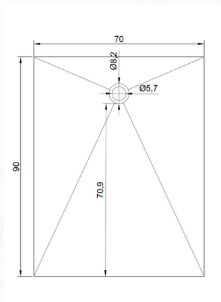
COD.PD_3 PIATTO DOCCIA 90X70 CON FORO ALTO
