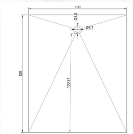
COD.PD_4 PIATTO DOCCIA 120X100 CON FORO ALTO
