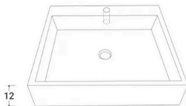
COD.LE 2 LAVABO 40X40 CM CON FORO MISCELATORE
